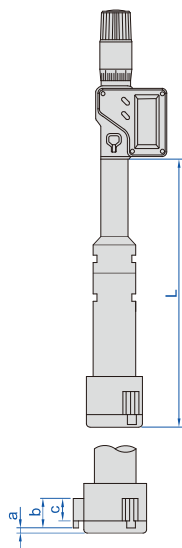
C型 12-50mm, 硬质合金测量面 三点式
