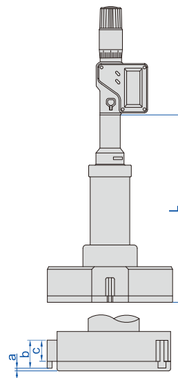
D型 50-300mm, 硬质合金测量面 三点式
